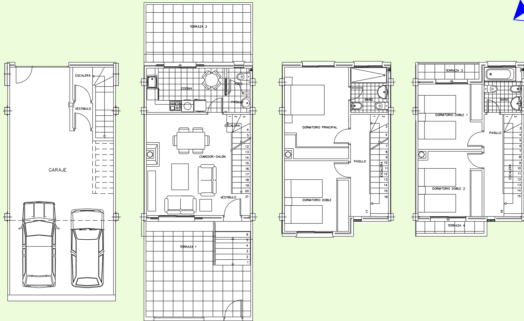
PLANTA SOTANO
